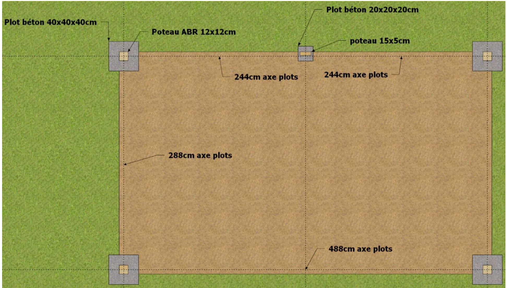
Position des blocs de bétons - Abrivert
